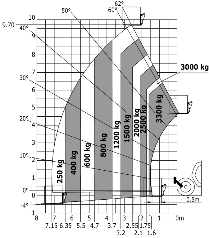
All terrein abacus (EN 1459 B)
